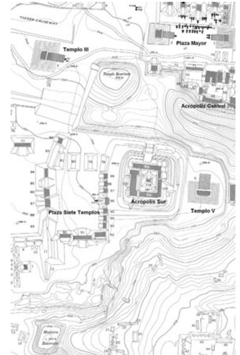
Figura 1: Planta de arquitectura del conjunto central.
